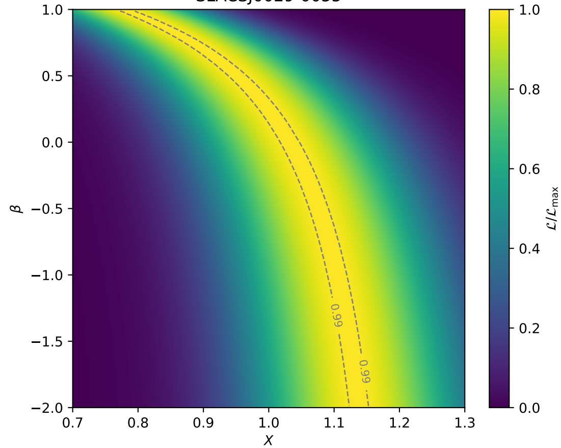
SLACSJ0029-0055
