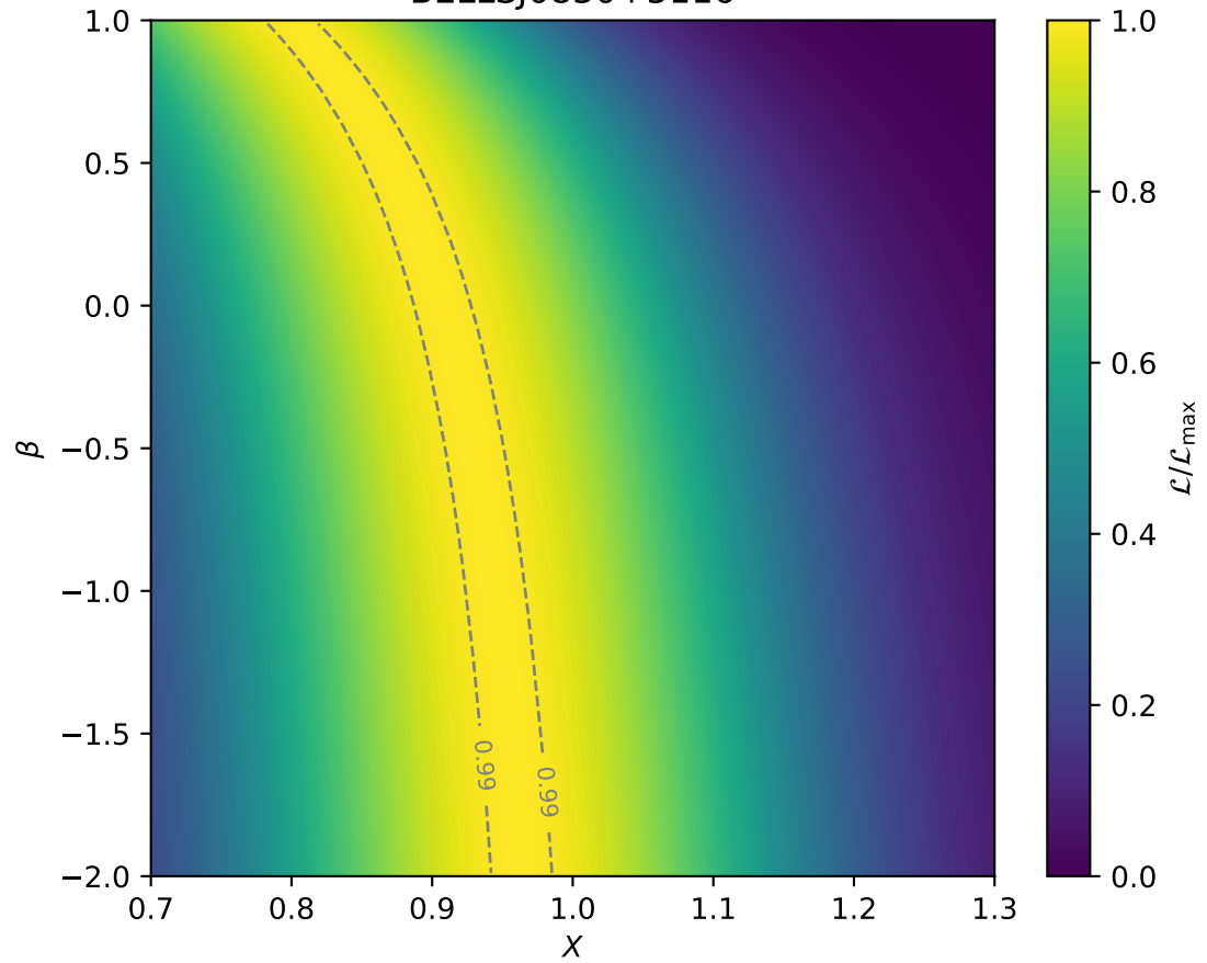
BELLSJ0830+5116
