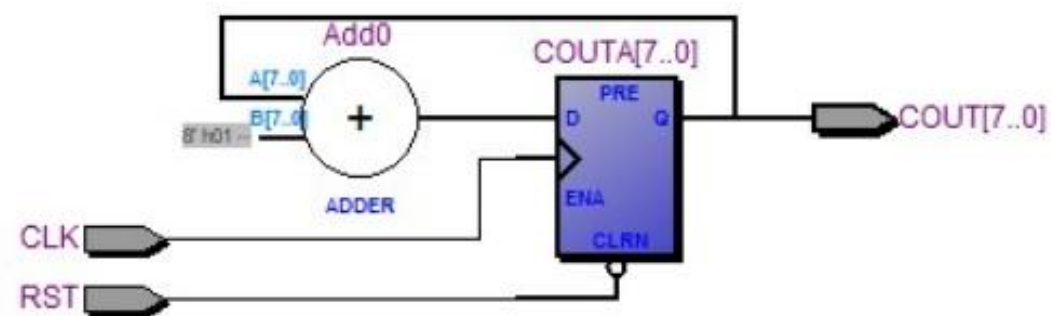
RTL结构图
