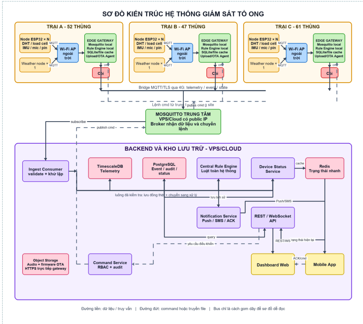
Hình 1. Sơ đồ kiến trúc hệ thống IoT của Hợp tác xã Ong Mật Cao Nguyên Xanh
