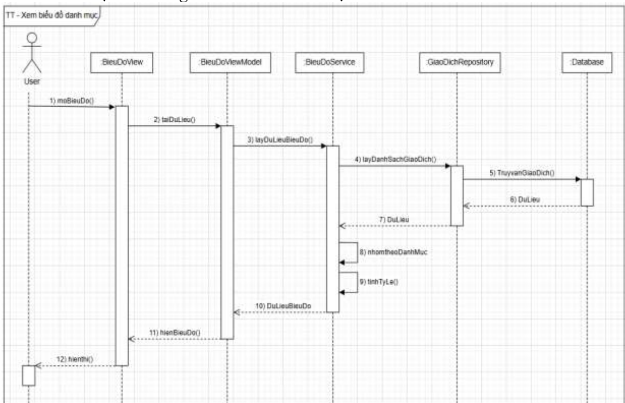
Hình 2.26 Biểu đồ tuần tự chức năng Xem biểu đồ danh mục
