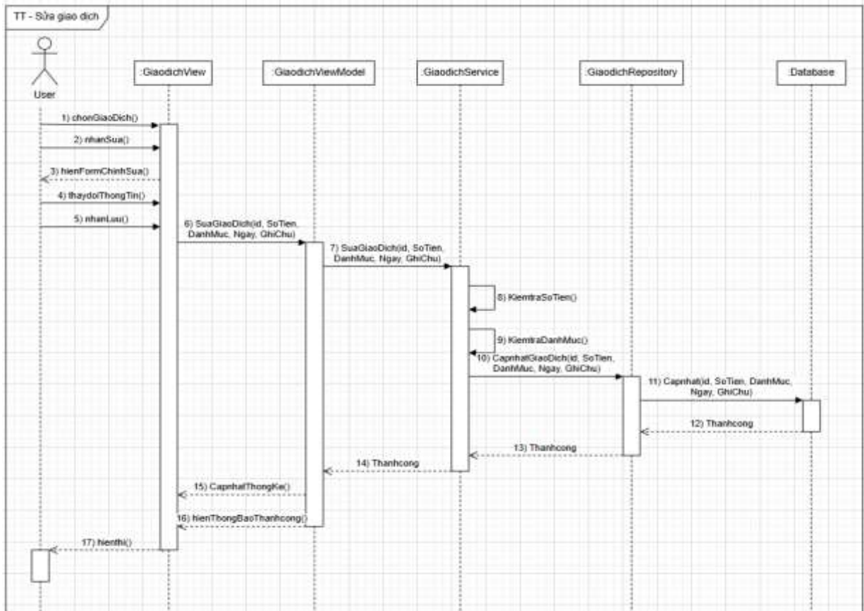
Hình 2.23 Biểu đồ tuần tự chức năng Sửa giao dịch
