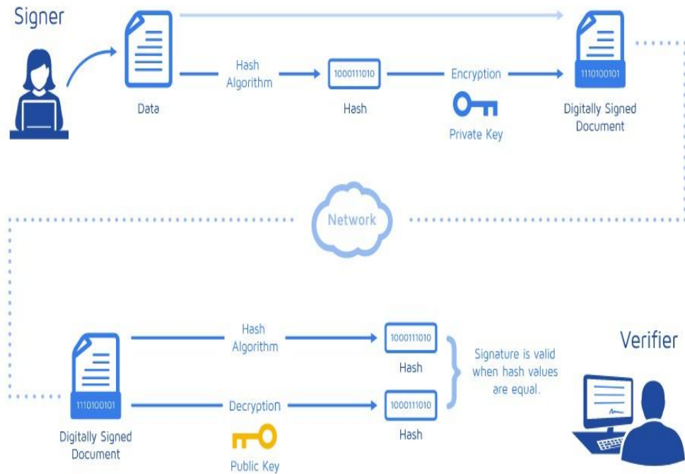
Hình 2.3. Quy trình tạo chữ ký số
