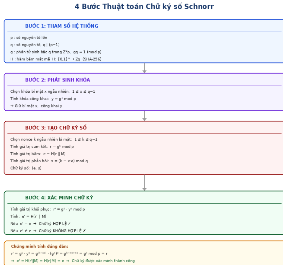
Hình 2.5. Lưu đồ 4 bước thuật toán chữ ký số Schnorr
