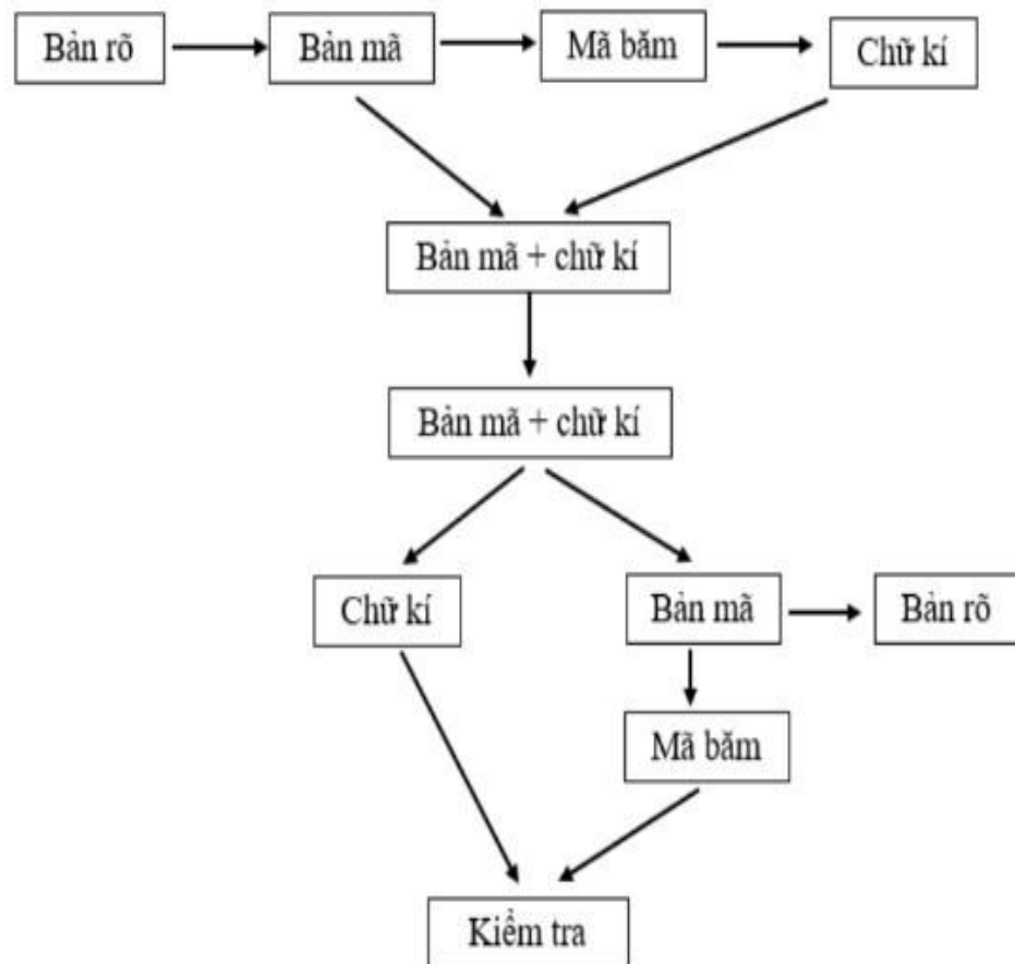
Hình 2.2. Sơ đồ chữ ký số
