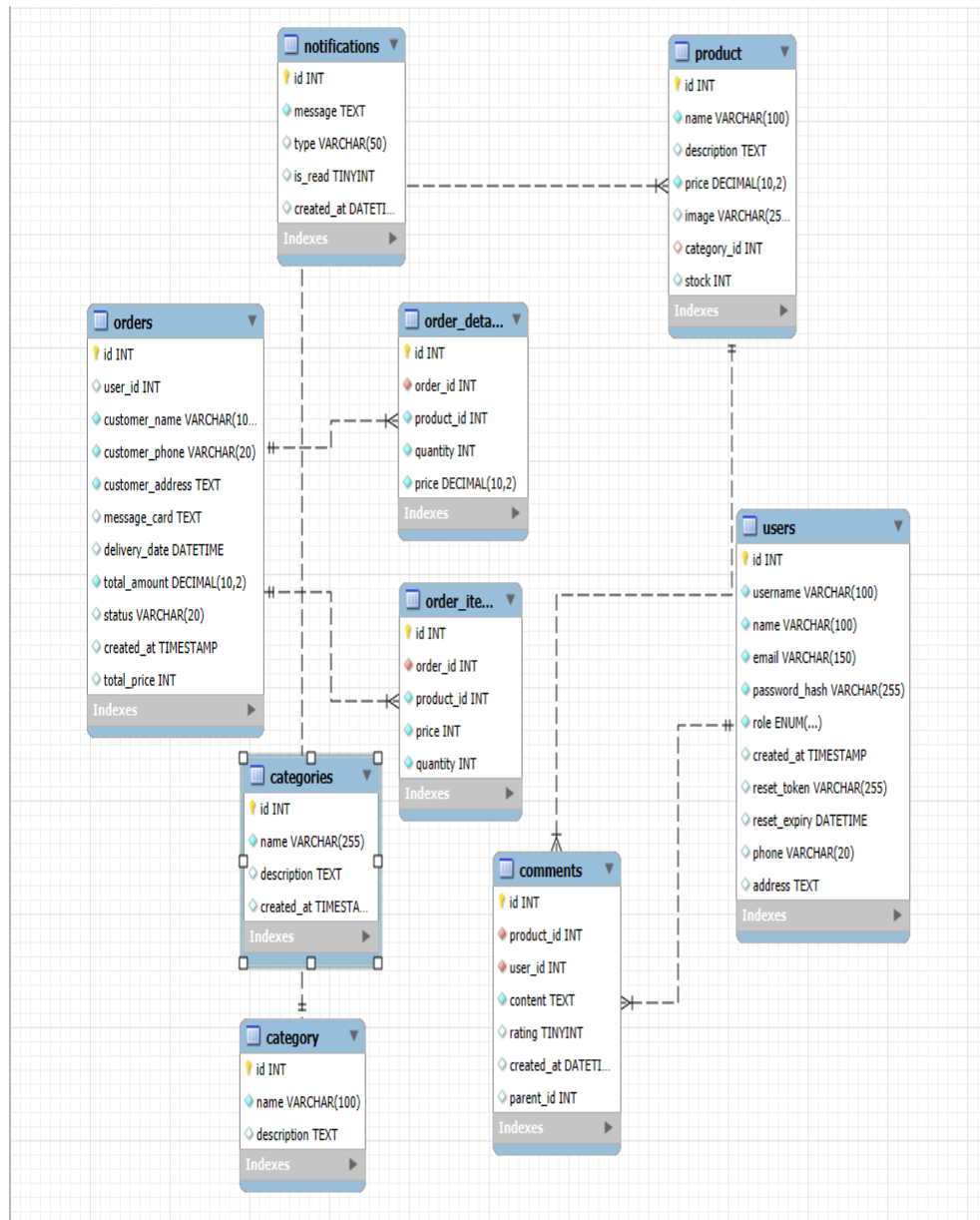
Hình 1: Sơ đồ thiết kế cơ sở dữ liệu
