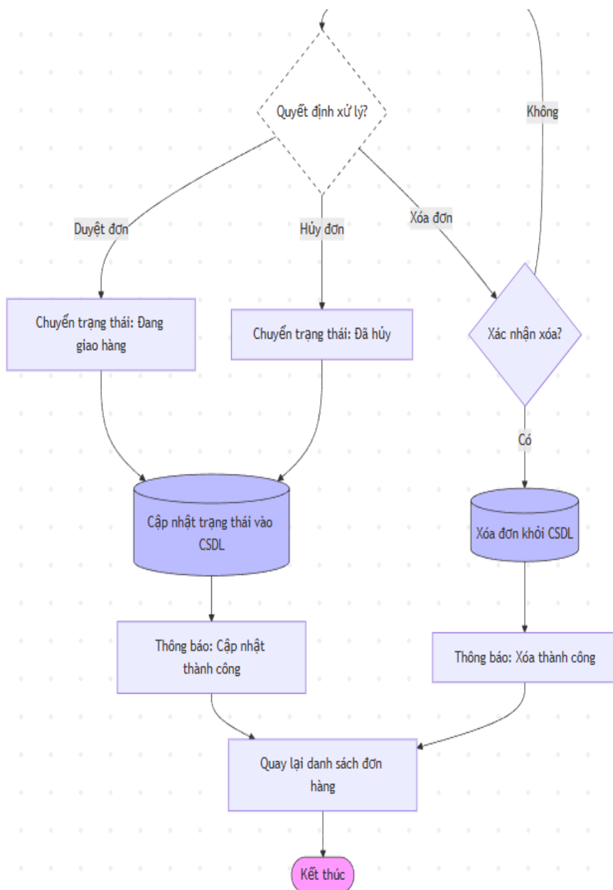
Hình 3: Sơ đồ luồng quy trình xử lý đơn hàng của Admin
