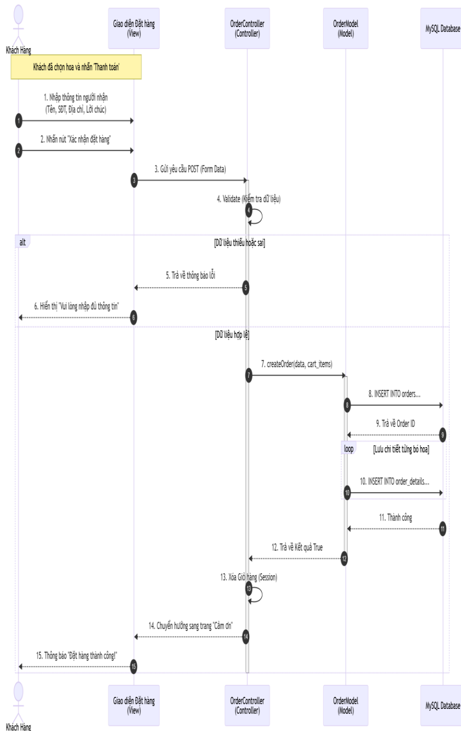
Hình 5: Sơ đồ tuần tự chức năng đặt hàng (user)
