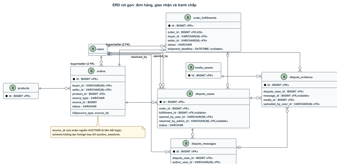
Hình 4.10: ERD rút gọn của nhóm đơn hàng, giao nhận và tranh chấp
