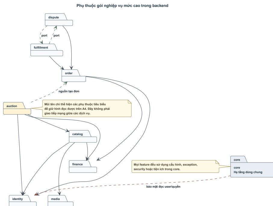
Hình 4.1: Phụ thuộc gói nghiệp vụ mức cao trong backend Nguồn: Tổng hợp từ quan hệ phụ thuộc trong backend.
