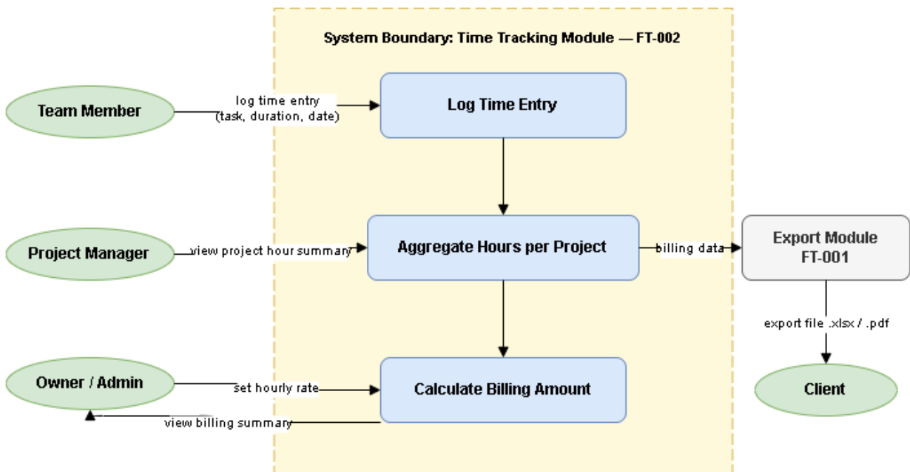
Context Diagram — Time Tracking Module (FT-002)
