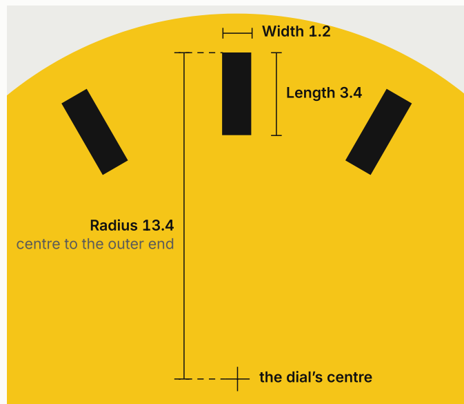
bar Length 3.4 · Width 1.2
