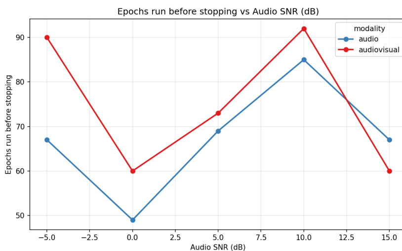
Σχήμα 31: Γράφημα αριθμού εποχών εκπαίδευσης για διάφορες τιμές audio SNR
