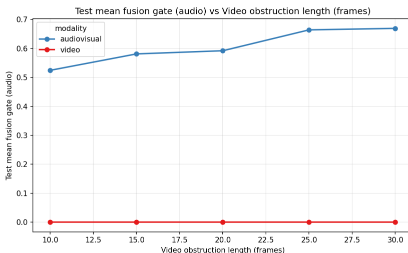
Σχήμα 43: Γράφημα τιμών της audio gate στο test set για διάφορες τιμές obstructed video frames
