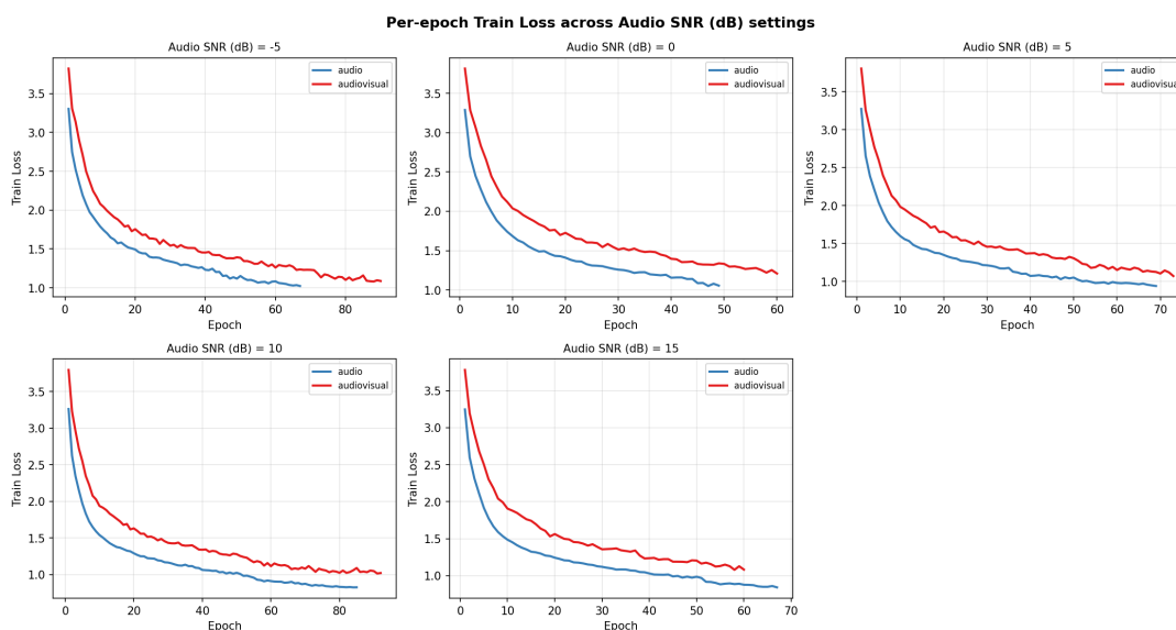
Σχήμα 26: Γραφήματα τιμών train loss per epoch για διάφορες τιμές audio SNR
