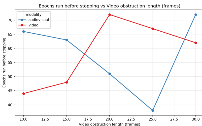
Σχήμα 42: Γράφημα αριθμού εποχών εκπαίδευσης για διάφορες τιμές obstructed video frames
