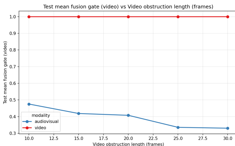
Σχήμα 44: Γράφημα τιμών της video gate στο test set για διάφορες obstructed video frames
