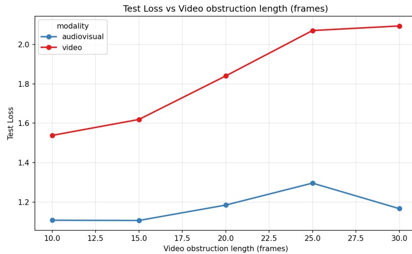
Σχήμα 45: Γράφημα τιμών της loss function στο test set για διάφορες τιμές obstructed video frames
