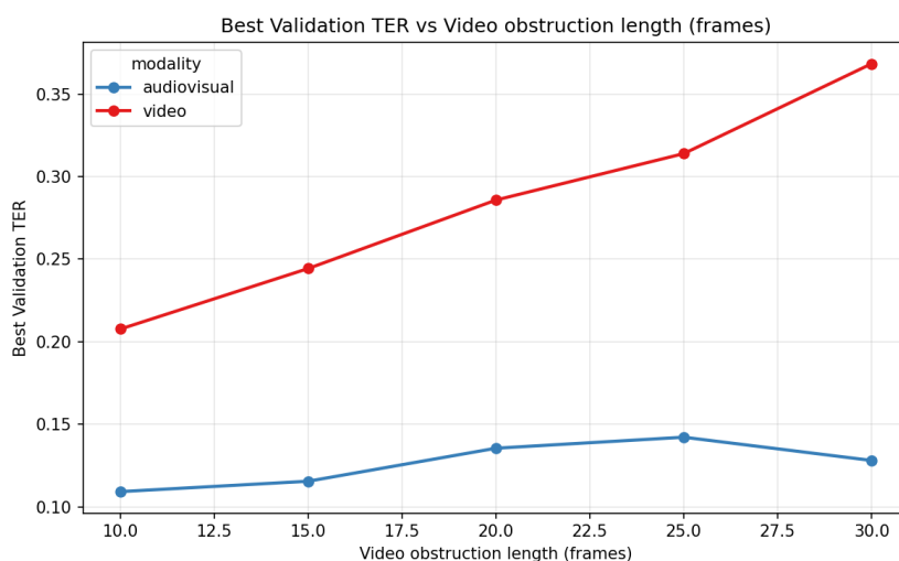
Σχήμα 36: Γράφημα τιμών του βέλτιστου val TER για διάφορες τιμές obstructed video frames
