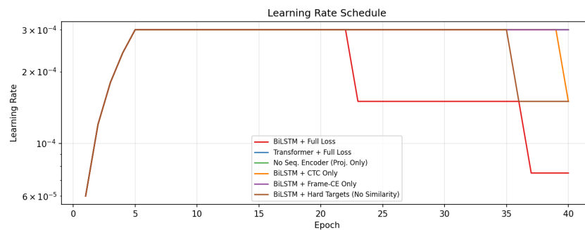
Σχήμα 19: Γράφημα τιμών του ρυθμού μάθησης (learning rate) για κάθε epoch
