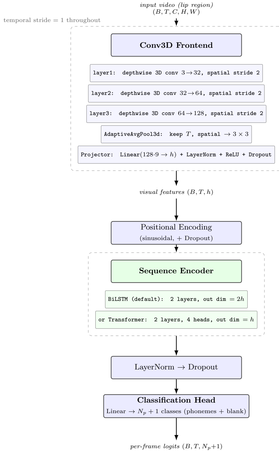
Σχήμα 6: Σχηματική παρουσίαση της προτεινόμενης μεθόδου
