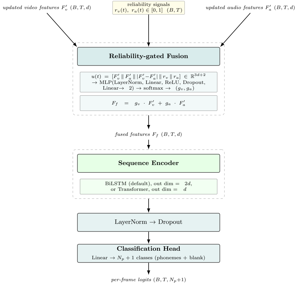
Σχήμα 8: Σχηματική παρουσίαση της προτεινόμενης μεθόδου για το audiovisual model, 2ο σχήμα
