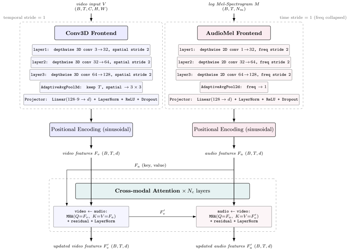
Σχήμα 7: Σχηματική παρουσίαση της προτεινόμενης μεθόδου για το audiovisual model, 1ο σχήμα
