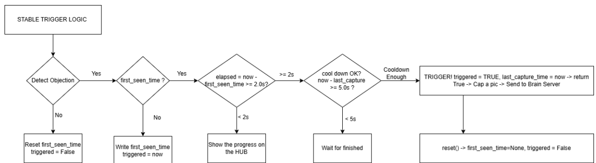
Hình 3.17: Lưu đồ giải thuật của thuật toán StableTrigger
