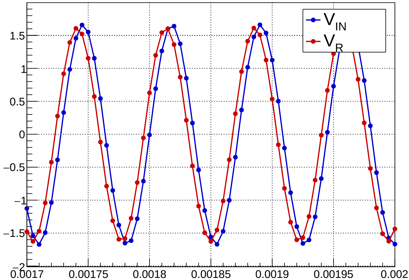
Ampiezza del voltaggio ai capi del generatore e della resistenza
