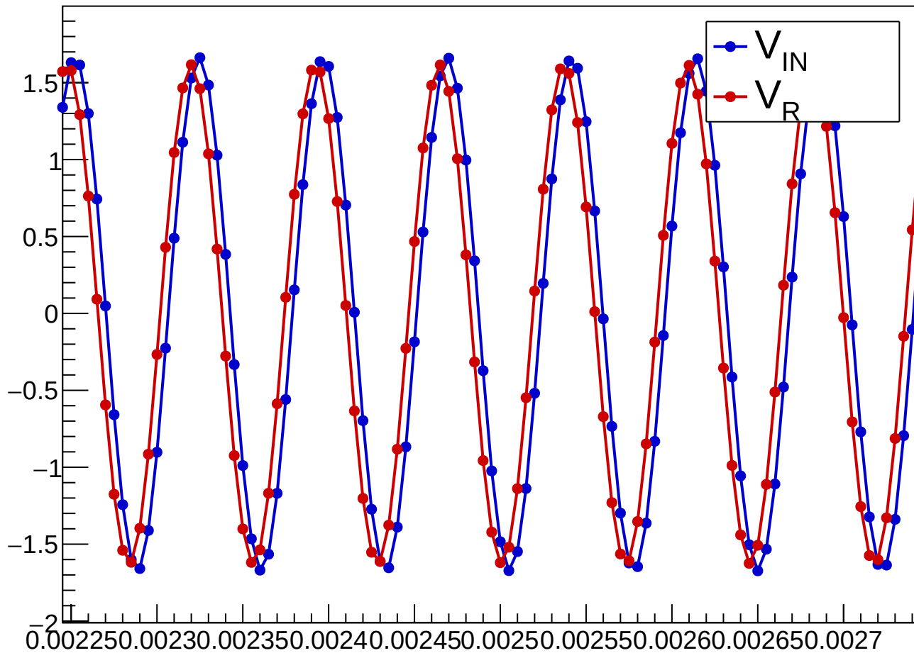
Ampiezza del voltaggio ai capi del generatore e della resistenza
