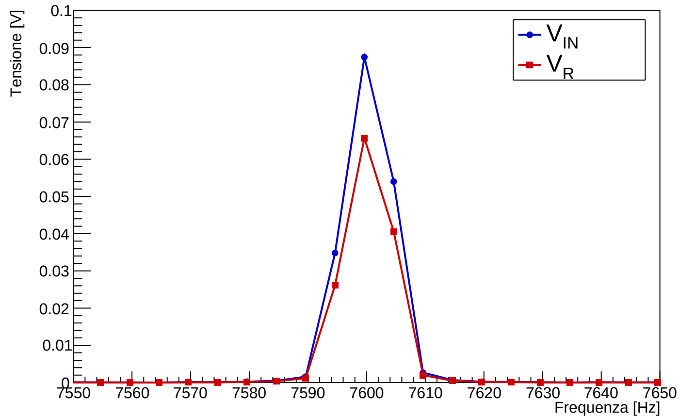
V_{IN} e V_R vs Frequenza
