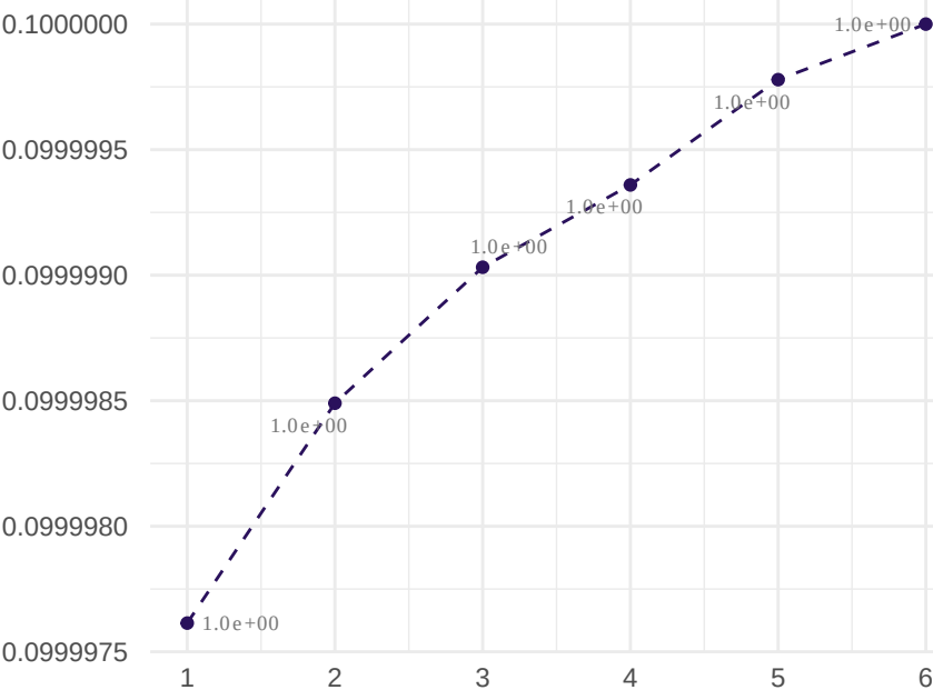
RsquaredSD
