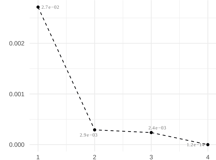
RMSESD
