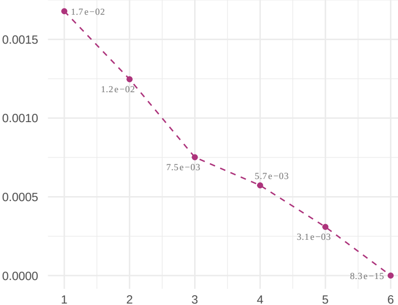
RMSESD
