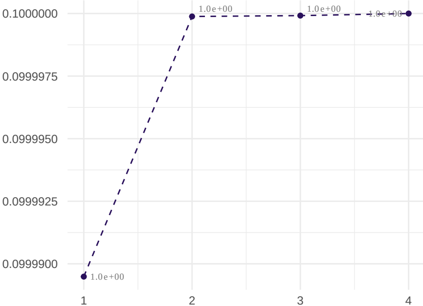
RsquaredSD
