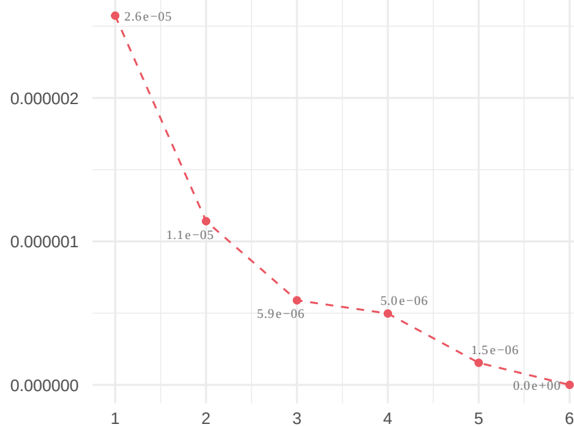
RsquaredSD
