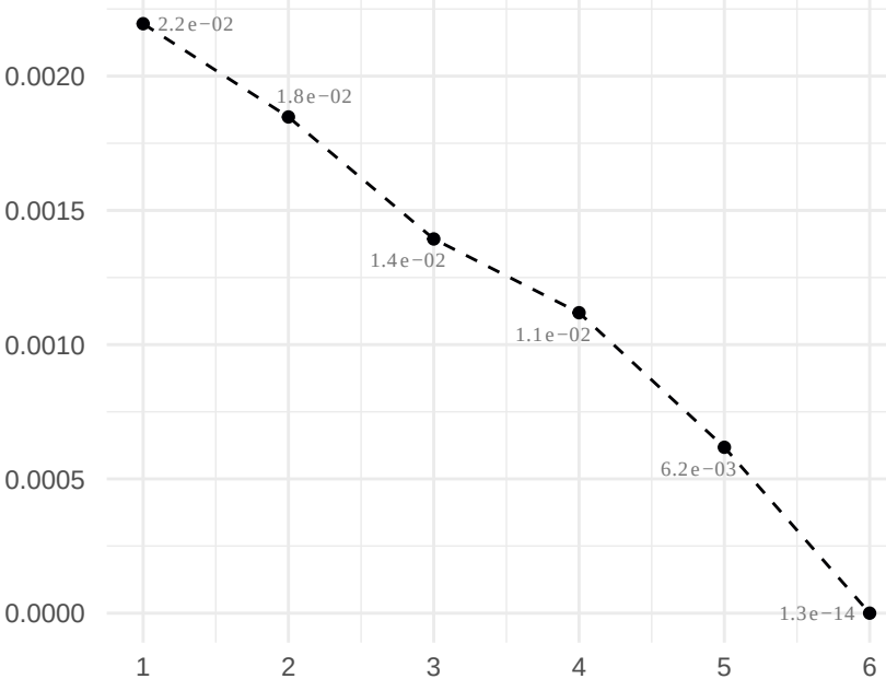
RMSESD
