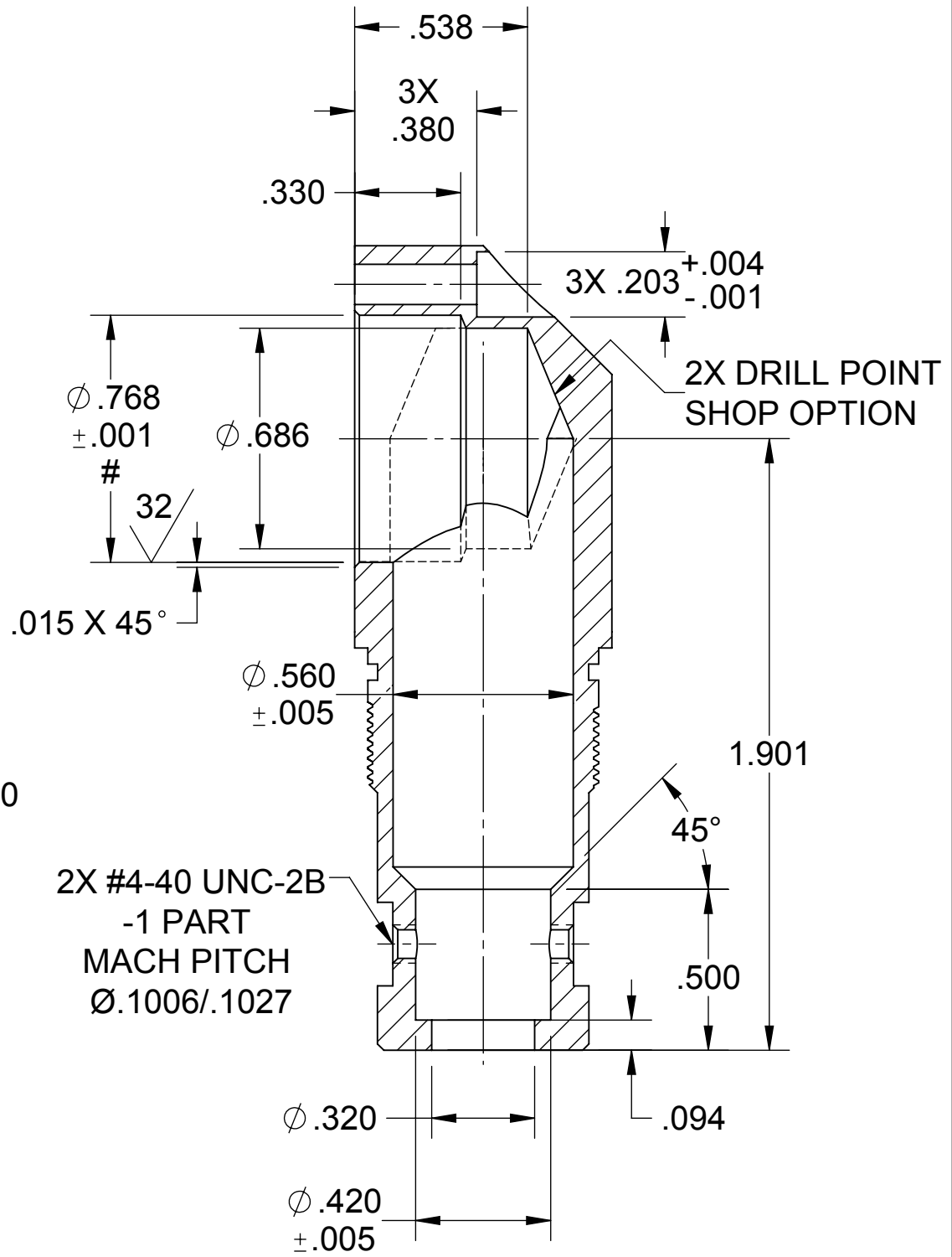
SECTION A-A
