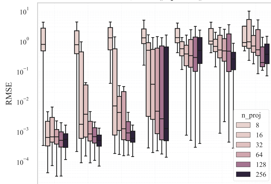
Velocity Error \|\mathbf{v}_0^* - \widehat{\mathbf{v}}_0\|_2
