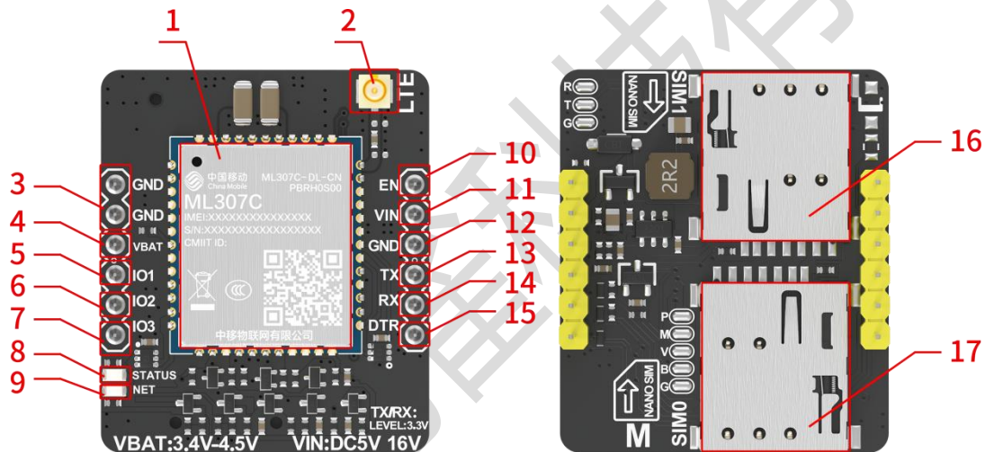
图 3：底板定义(CT12-B)
