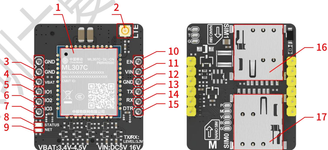
图 4：底板定义(CT12-C)
