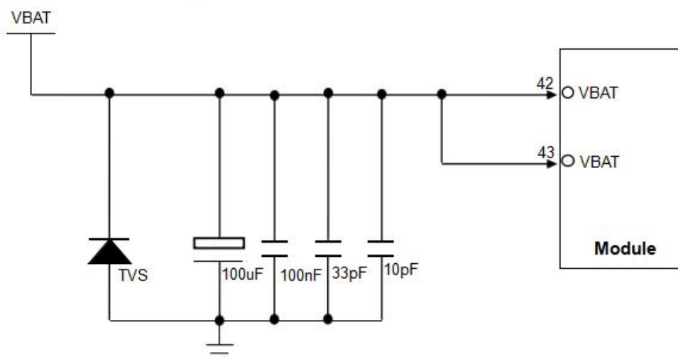
图 6：电池供电参考电路( CT12-C 模块 )
