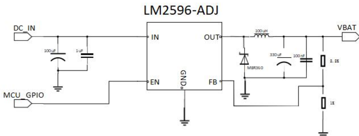
图 5：DC/DC 供电参考电路( CT12-B 模块 )
