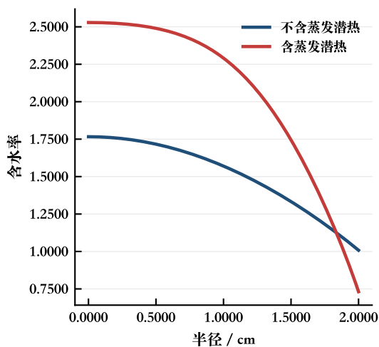
(d) 末时刻含水率径向剖面
