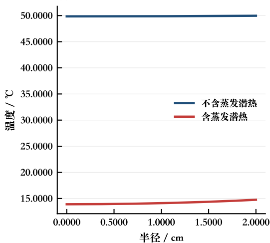
(c) 末时刻温度径向剖面
