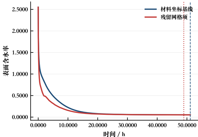
(c) 表面含水率演化
