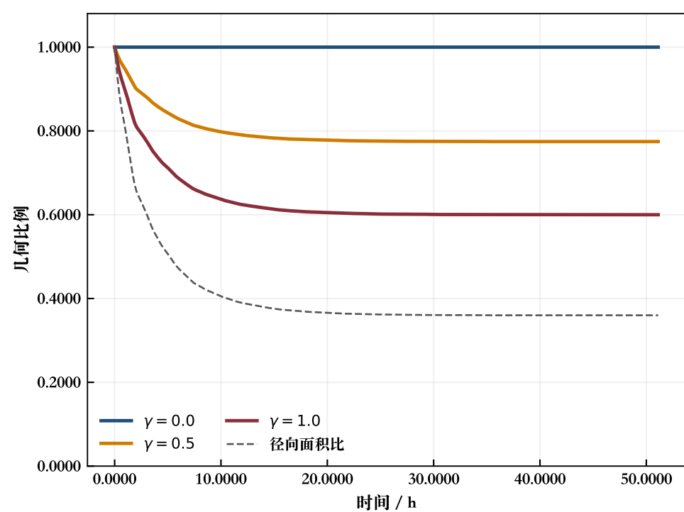
(a) 轴向长度收缩对几何比例的影响
