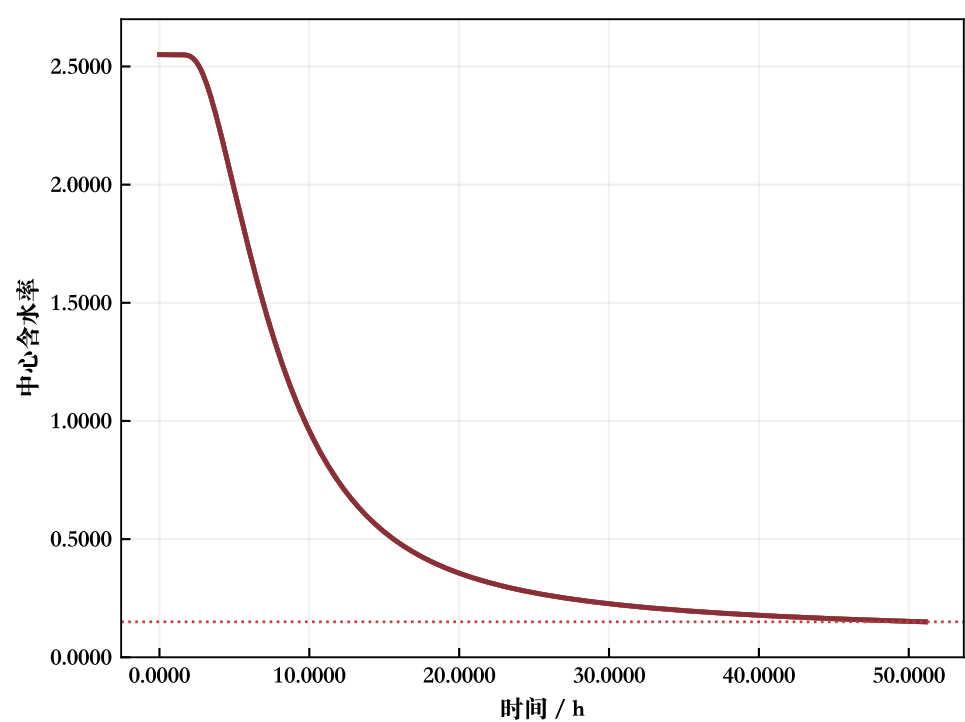
(b) 不同伽马下中心含水率等价性
