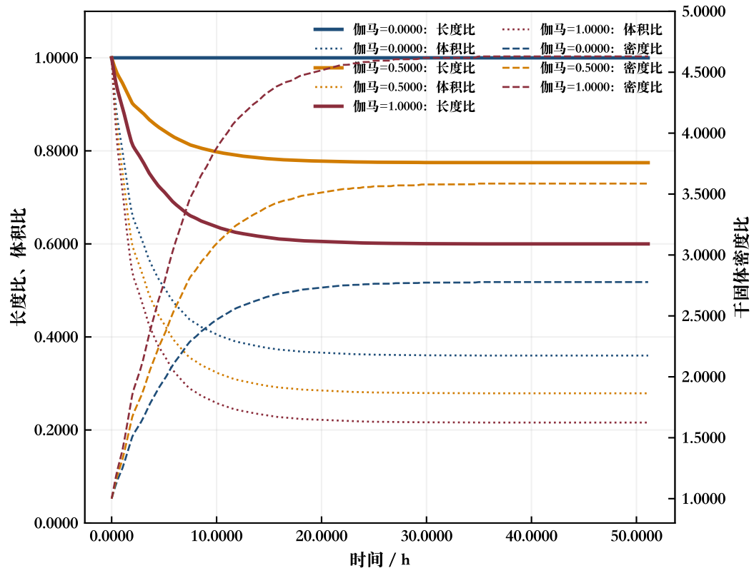
(b) 几何诊断: 长度、体积与干固体密度比例
