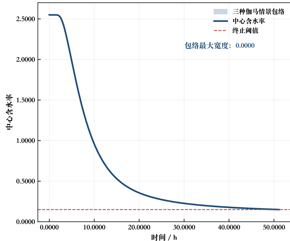
(a) 场变量等价性: 中心含水率上下浮动带
