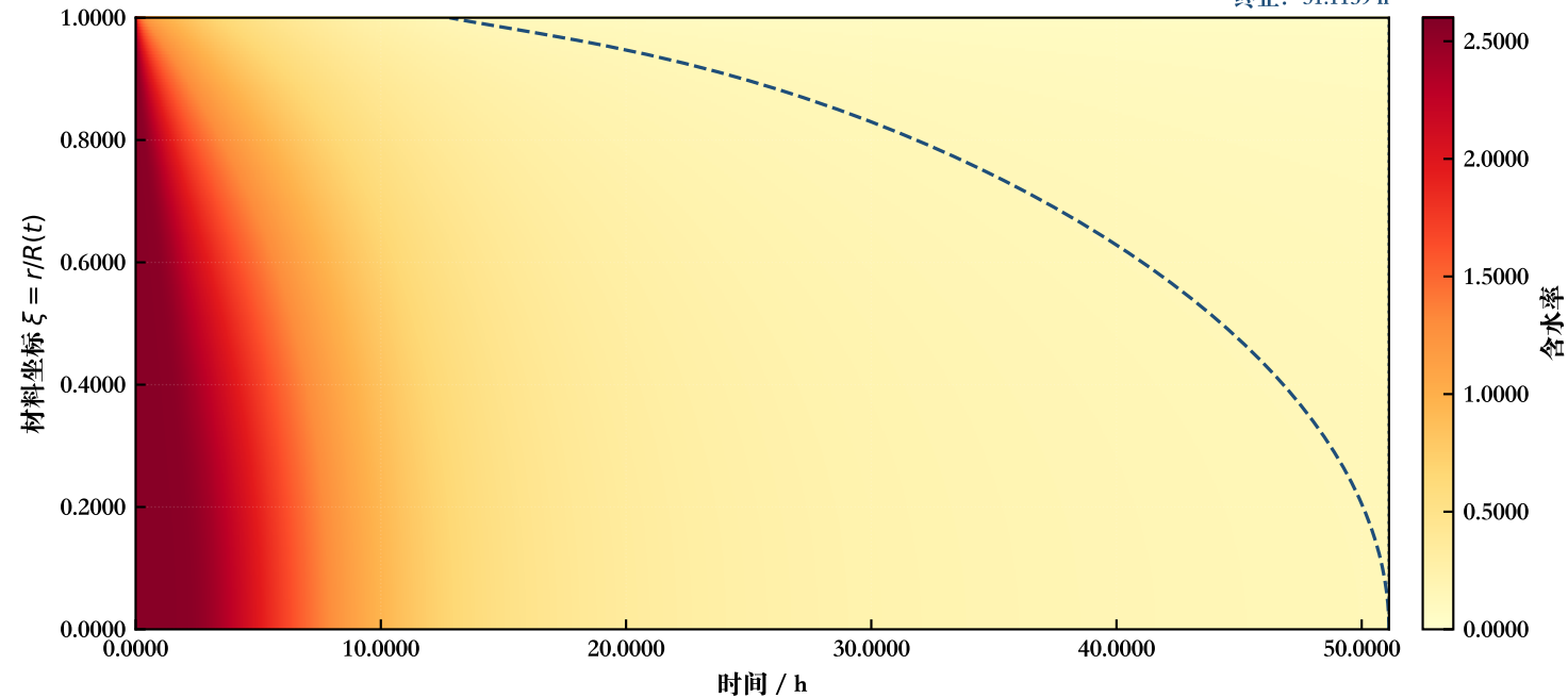
问题四基线的材料坐标含水率时空演化
