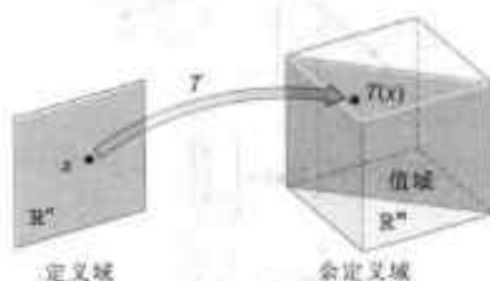
图 1-35 T: \mathbb{R}^n \rightarrow \mathbb{R}^m 的定义域、余定义域和值域
