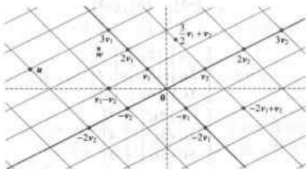
图 1-14 v_1 与 v_2 的线性组合
