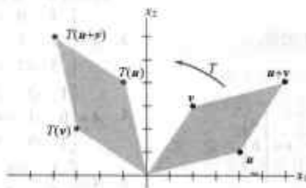
图 1-39 旋转变换
