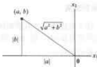
图 6-1 \|v\| 作为长度的几何意义
