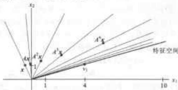
图 5-26 由 x, Ax, A^2x, \cdots, A^7x 确定的方向
