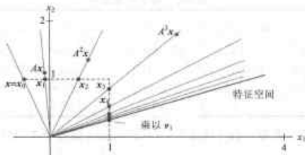
图 5-27 x, Ax, A^2x, \dots, A^kx 的倍乘
