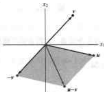
图 1-13 向量减法
