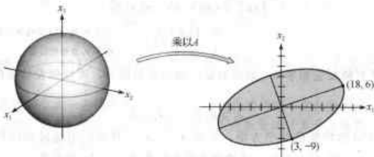
图 7-13 从 \mathbb{R}^3 到 \mathbb{R}^2 的一个变换
