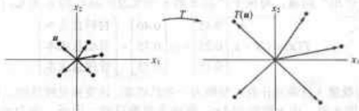
图 1-38 拉伸变换
