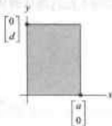
图 3-2 面积 = |ad|
