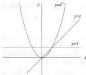
图 4-14 P_3 的标准基
