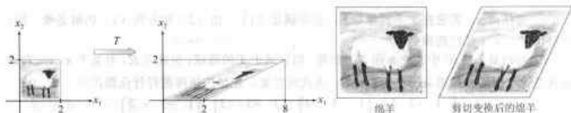
图 1-37 剪切变换
