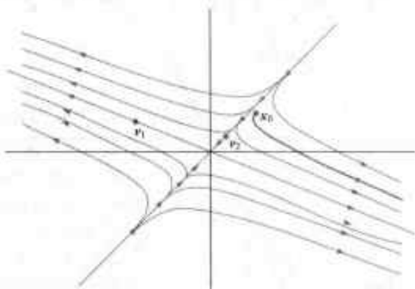
图 5-23 原点是鞍点
