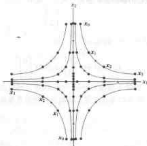
图 5-18 原点是鞍点
