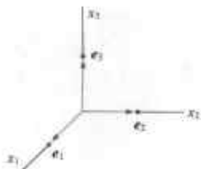
图 2-27 \mathbb{R}^3 的标准基
