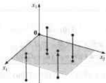
图 1-36 投影变换
