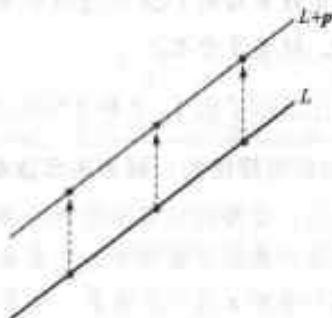
图 1-24 直线的平移
