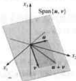
图 1-17 \text{Span}\{u, v\} 是通过原点的平面
