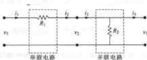
图 2-14 梯级电路
