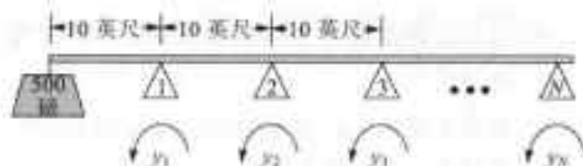
图 4-32 悬梁上的弯矩
