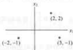
图 1-7 用点表示向量
