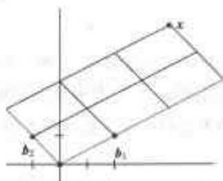
图 4-18 x 的 B -坐标向量为 (3, 2)
