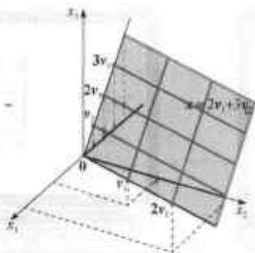
图 4-21 \mathbb{R}^3 中平面 H 上的坐标系
