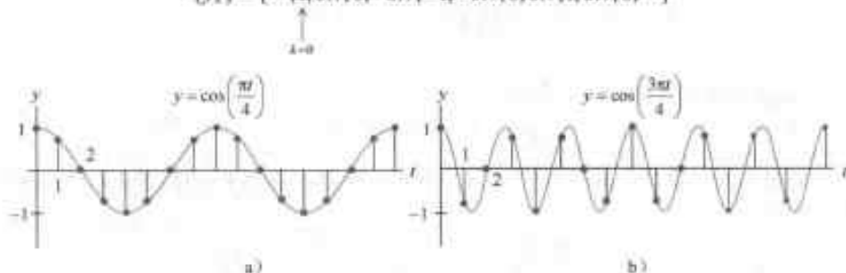
图 4-30 具有不同频率的离散信号
