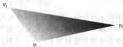
图 8-11 插入颜色
