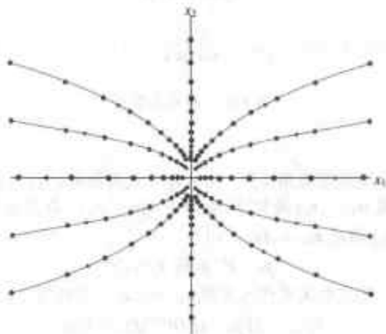
图 5-17 原点排斥子
