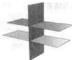
d) 三个平面没有交点
