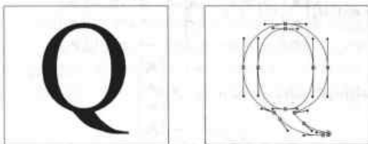
图 8-38 PostScript 字符
