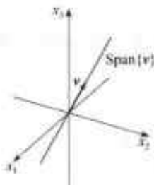
图 1-16 \text{Span}\{v\} 是通过原点的直线
