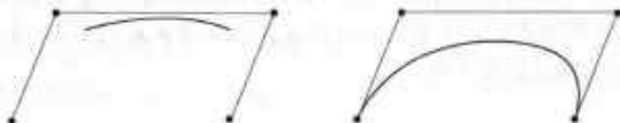
图 8-43 B-样条线段和贝塞尔曲线
