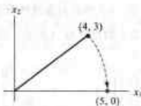
图 1-49 \mathbb{R}^2 中的吉温斯旋转
