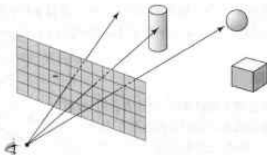
图 8-12 从眼睛通过屏幕到最近物体的射线
