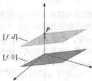
图 8-17 平行超平面, f(p)=d
