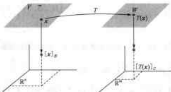
图 5-6 V 到 W 的线性变换
