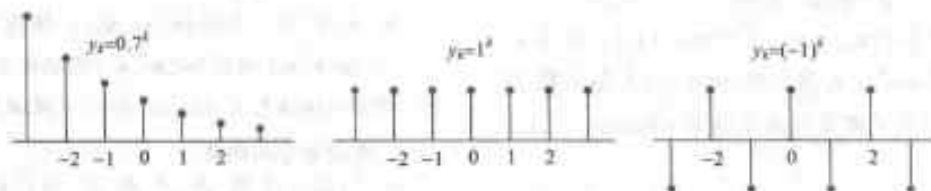
图 4-27 S 中三个信号
