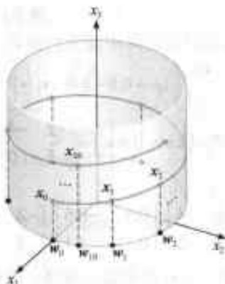
图 5-15 点 w_0 和 x_0 在有复特征值的 3 \times 3 矩阵作用下的迭代
