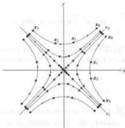
图 5-19 原点是鞍点
