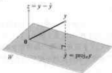
图 6-18 y 在 W 上的正交投影
