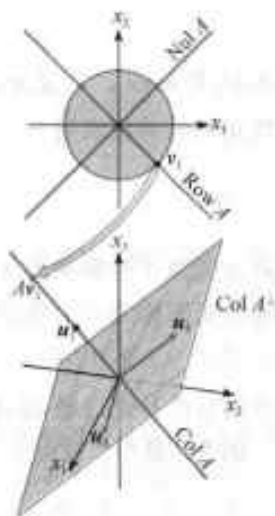
图 7-16 例 6 中的基本子空间
