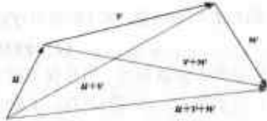
图 4-4 (u+v)+w=u+(v+w) ■
