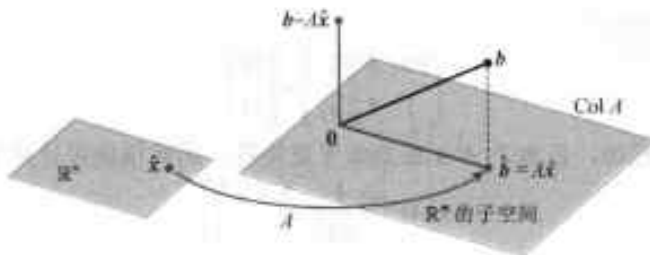
图 6-24 \mathbb{R}^n 中的最小二乘解 \hat{x}
