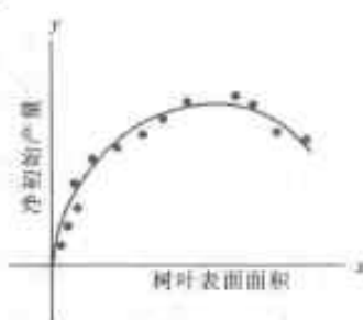
图 6-29 营养成分的产量
