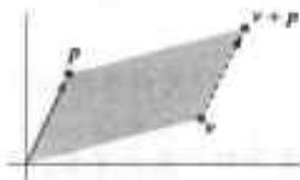
图 1-23 v 加上 p , 使 v 平移到 v + p
