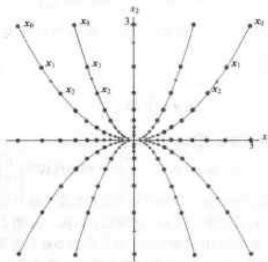
图 5-16 原点是吸引子
