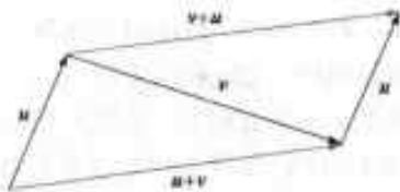
图 4-3 u+v=v+u
