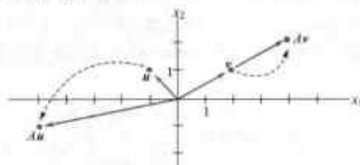
图 5-1 乘以 A 的作用
