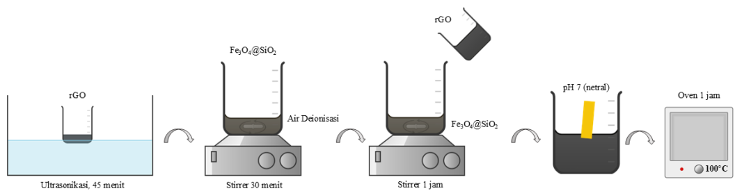
Gambar 4. Sintesis \text{Fe}_3\text{O}_4/\text{SiO}_2/\text{rGO} menggunakan pencampuran basah.
