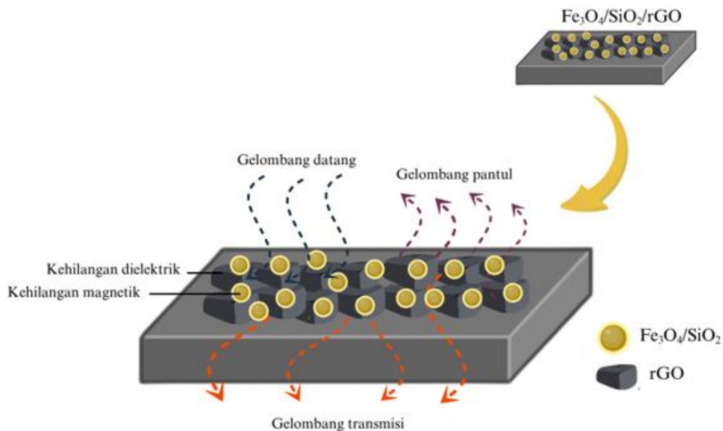
Gambar 11. Ilustrasi mekanisme penyerapan gelombang elektromagnetik \text{Fe}_3\text{O}_4/\text{SiO}_2/\text{rGO} .
