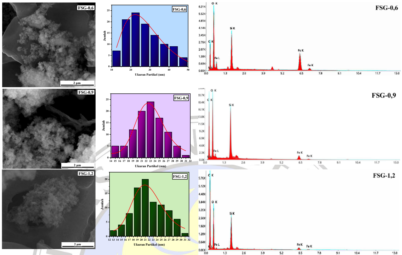
Gambar 9. Morfologi dan ukuran partikel \text{Fe}_3\text{O}_4/\text{SiO}_2/\text{rGO} .
