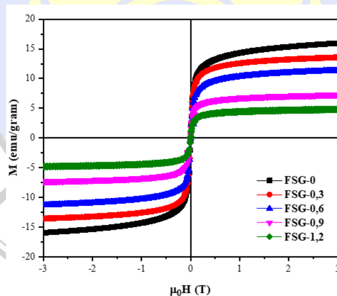
Gambar 10. Kurva histeresis dari nanokomposit \text{Fe}_3\text{O}_4/\text{SiO}_2/\text{rGO} .
