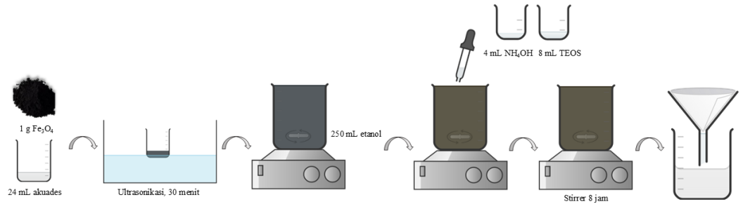
Gambar 3. Sintesis \text{Fe}_3\text{O}_4/\text{SiO}_2 menggunakan metode in-situ .
