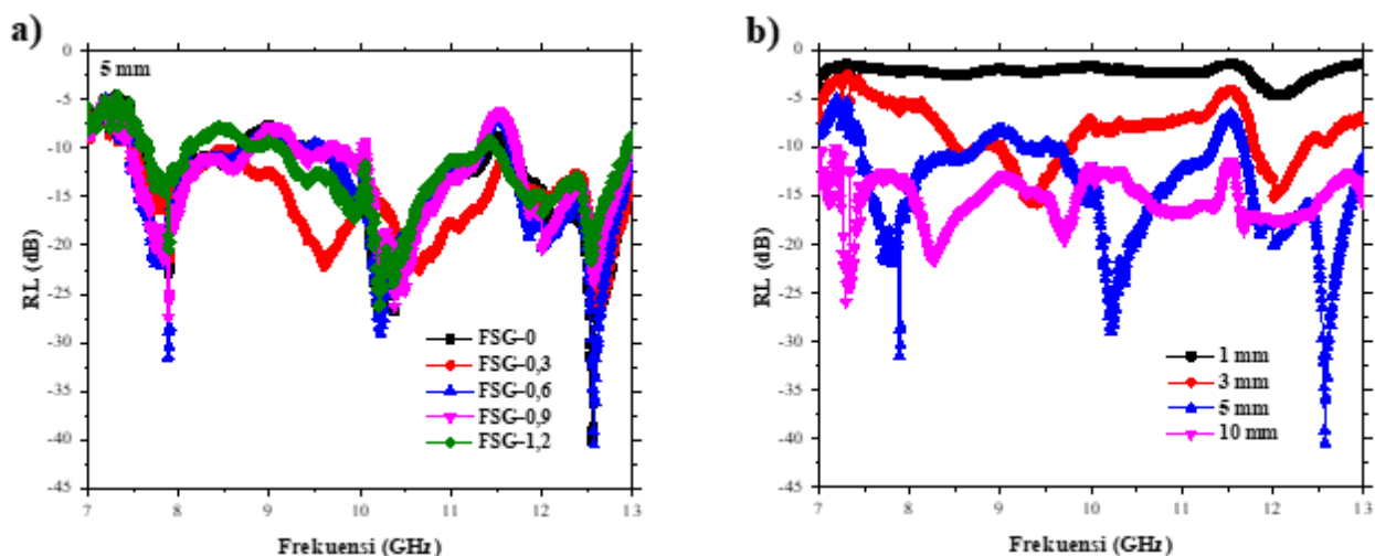
Gambar 15. Kurva RL Fe 3 O 4 /SiO 2 /rGO di a) 5 mm dan b) FSG-0,6.
