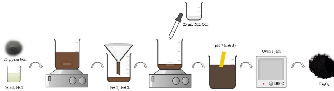
Gambar 2. Sintesis \text{Fe}_3\text{O}_4 dengan kopresipitasi.
