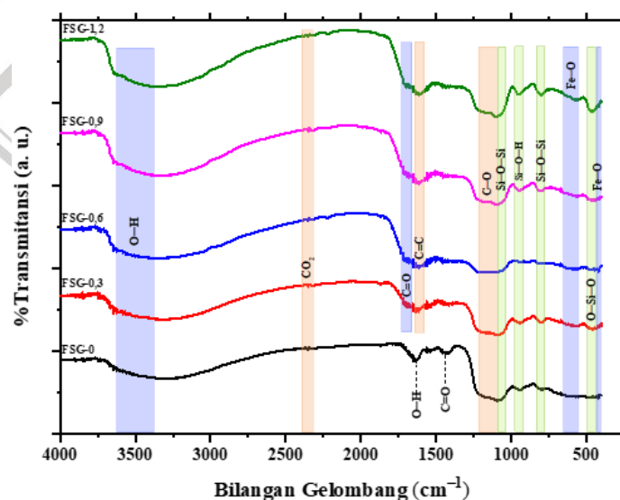
Gambar 8. Spektrum FTIR dari nanokomposit \text{Fe}_3\text{O}_4/\text{SiO}_2/\text{rGO} .
