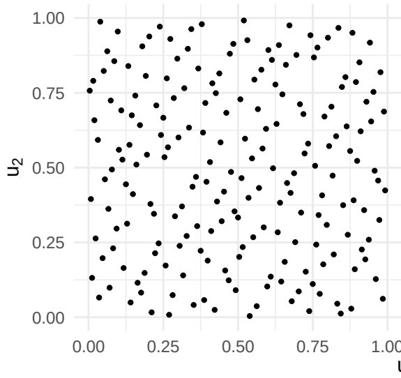
Halton
