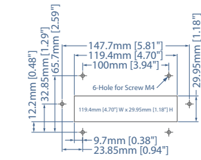
Cutout Dimensions
