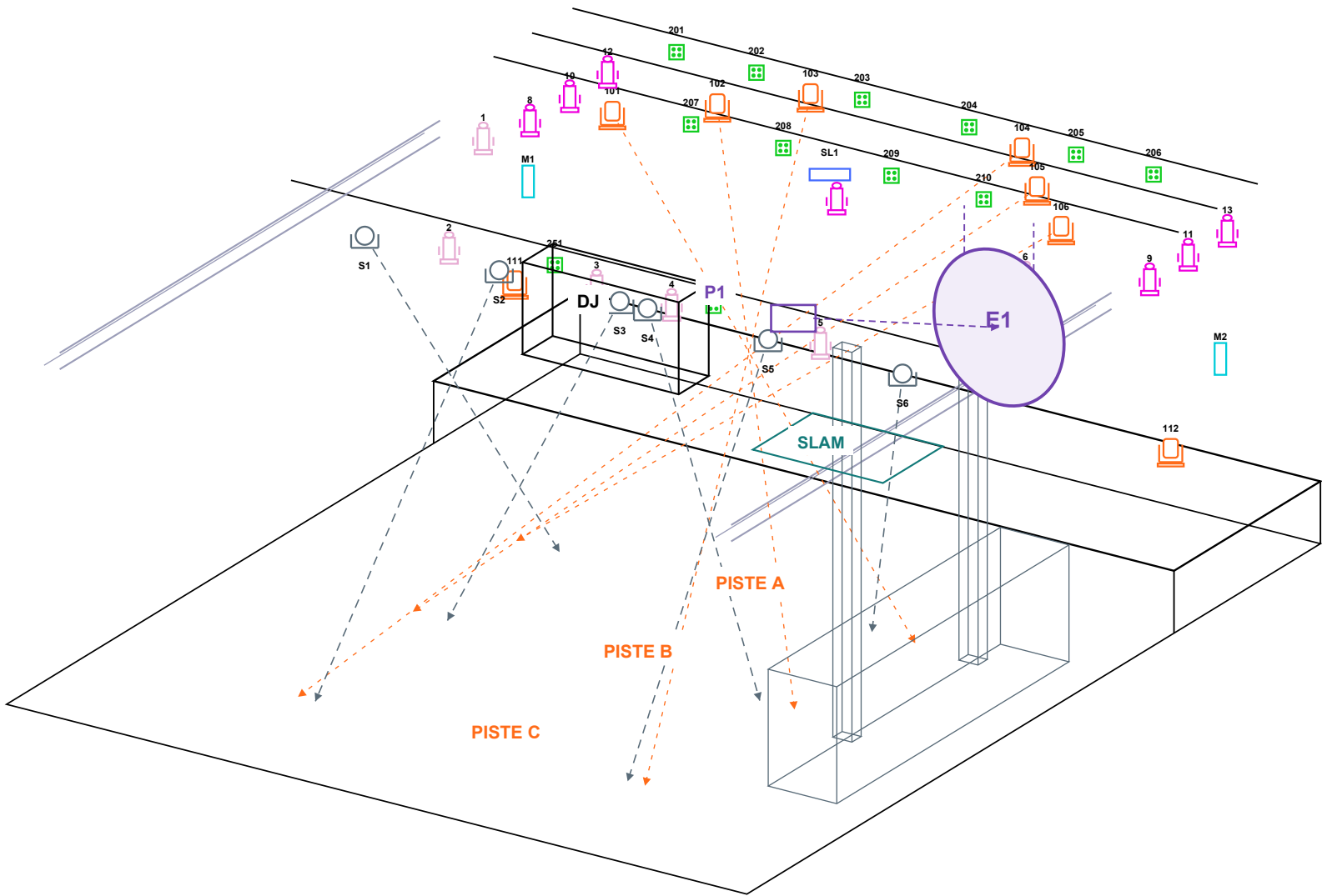
S1-S6 : 6 PAR proposés au-dessus de la piste. Les autres appareils conservent les positions du plan LX existant.
