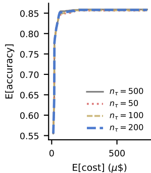
MMLU
