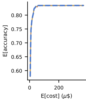
TriviaQA
