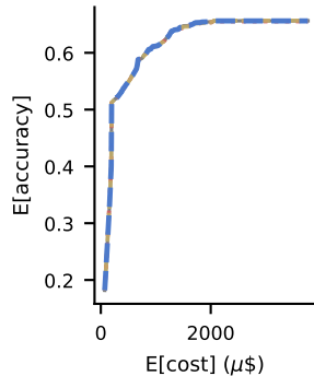
LiveCodeBench
