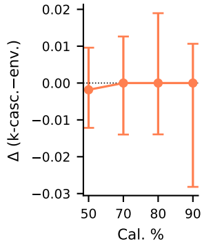
LiveCodeBench
