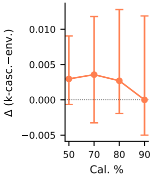
TriviaQA
