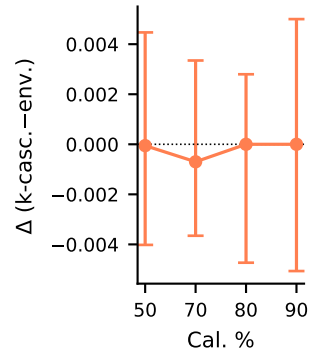
MMLU
