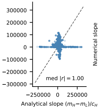
MMLU
