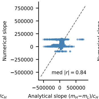
TriviaQA
