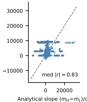
LiveCodeBench
