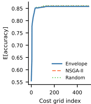
MMLU
