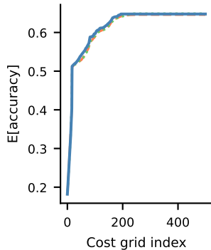
LiveCodeBench
