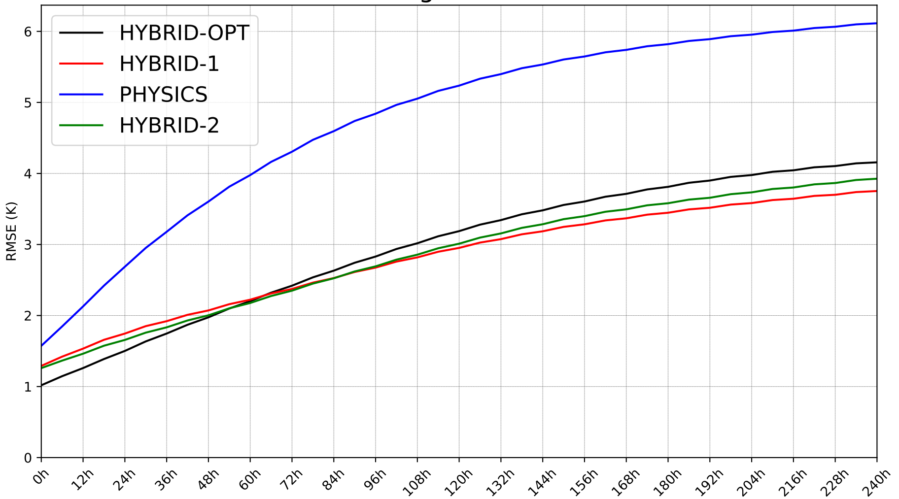
Sigma 0.51
