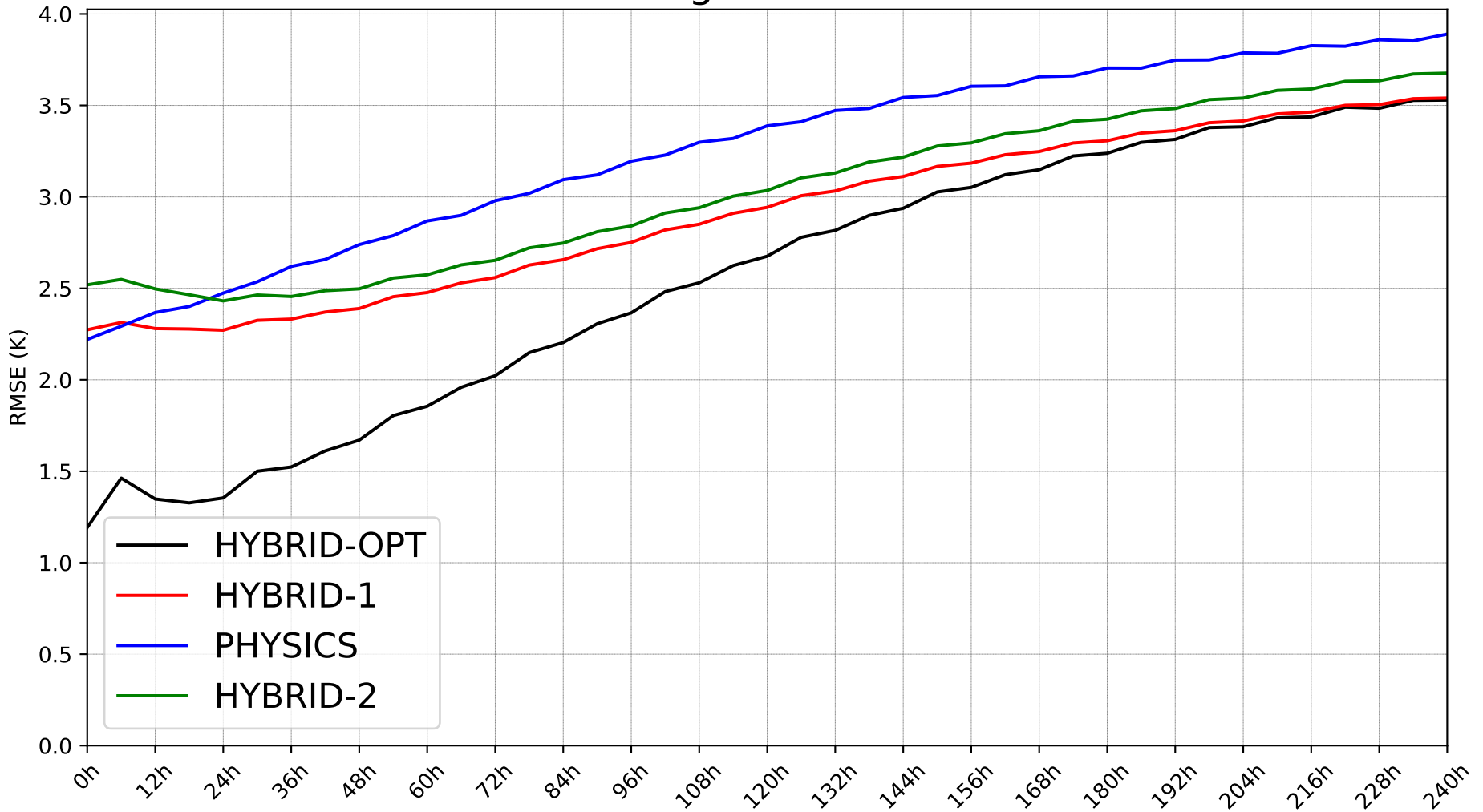
Sigma 0.95
