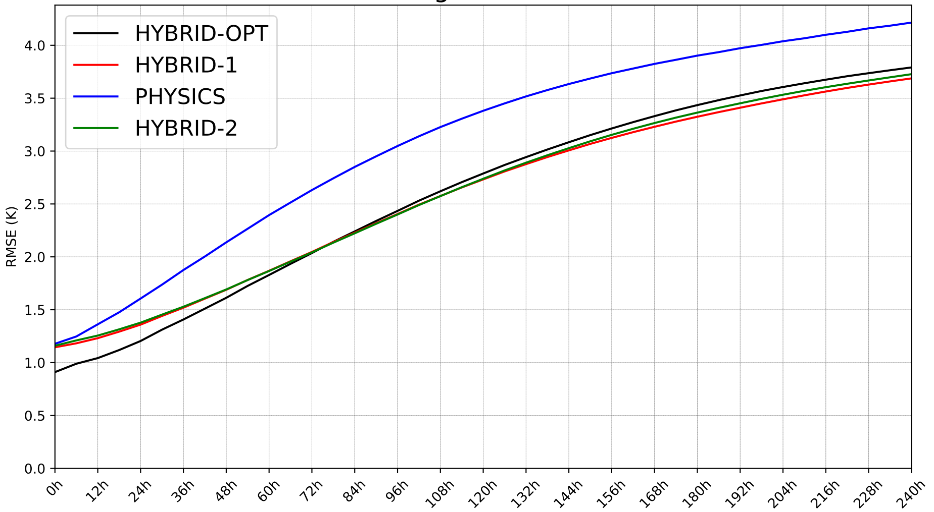
Sigma 0.95
