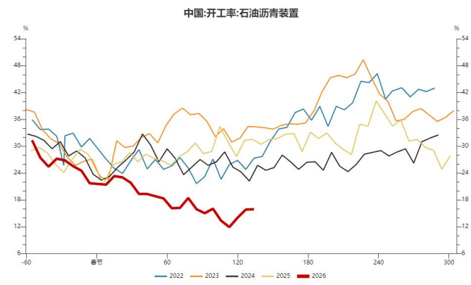
图 18： 沥青开工率上升
