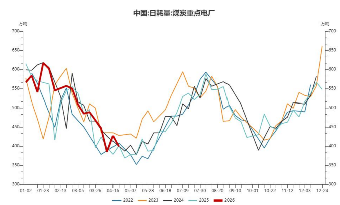
图 14：电厂日耗煤量下降
