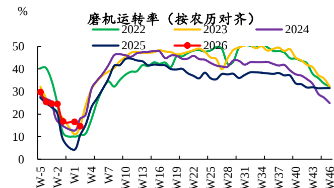
图3：磨机运转率高于 2025 年农历同期
