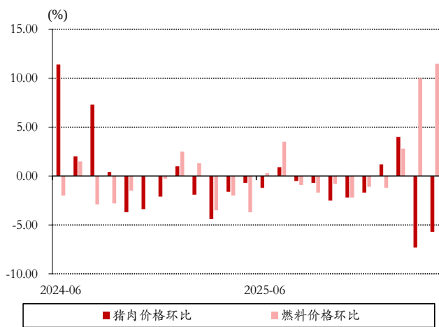
图表 5. 猪肉价格和燃料价格环比增速
