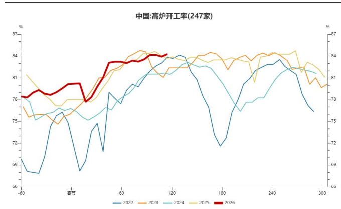
图 14：高炉开工率上升
