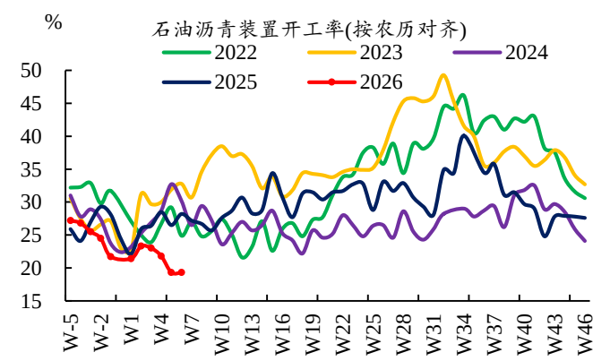
图2：石油沥青装置开工率逆季节性下行
