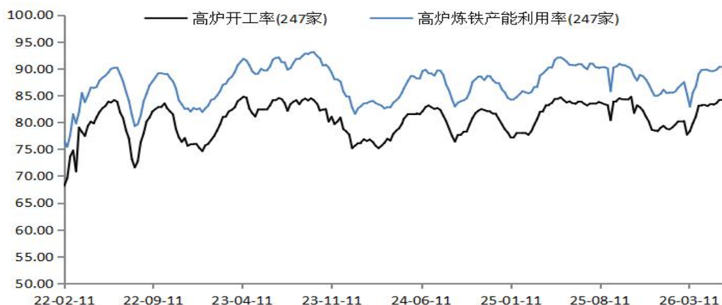
图表 1：钢厂高炉开工率和炼铁产能利用率
