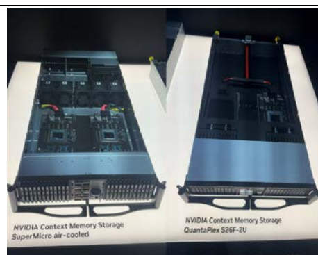
圖 7: 用於 BF 4 STX 的托盤級設計 (水冷和氣冷)
