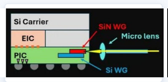
COUPE-EC
