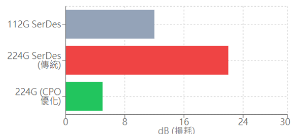
圖 1 電氣互連訊號損耗
