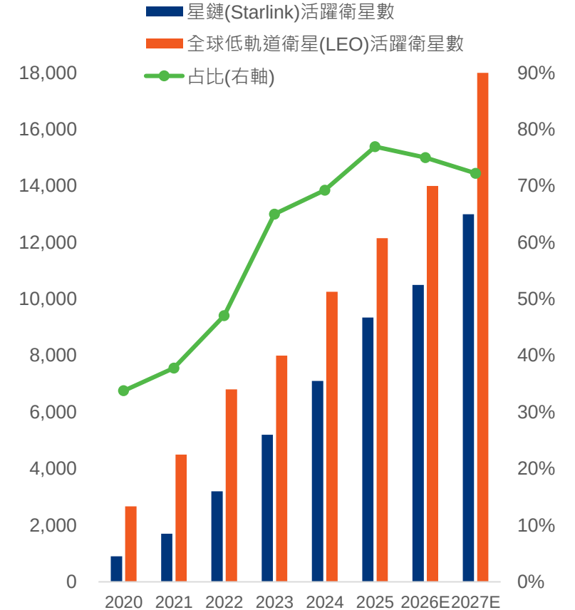
活躍衛星數量，個數
