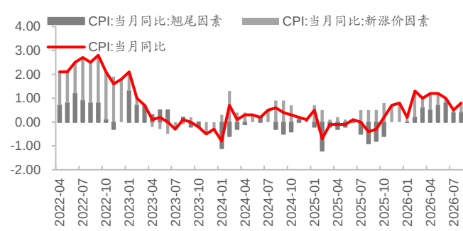
图2 8月CPI增速回升(%)
