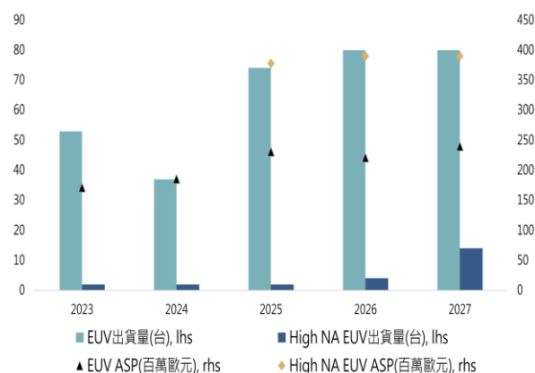
圖三：High NA EUV 將逐步放量
