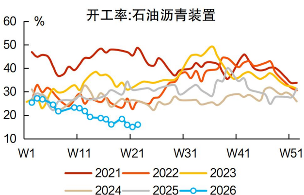
图表 8：高油价约束石油沥青开工率
