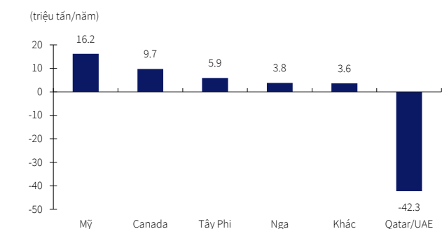
Biểu đồ 14. Dự báo thay đổi nguồn cung LNG 2026 (triệu tấn/năm)
