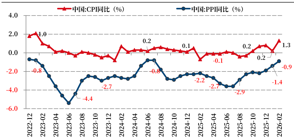
图 10：物价水平
